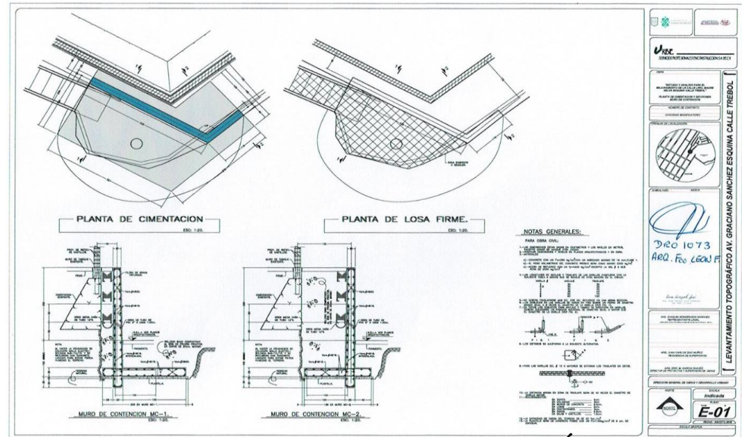
PROYECTO DE MURO DE CONTENCIÓN
